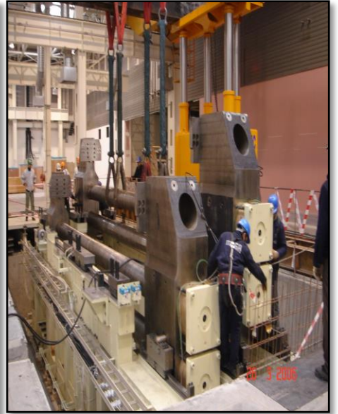
Enjeksiyon Makinası
